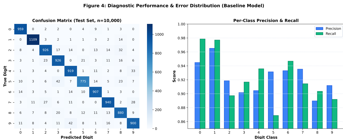
รูปที่ 4: Diagnostic Performance & Error Distribution (Baseline Model): ซ้าย: Heatmap เมตริกซ์ความสับสน ขวา: แผนภูมิแท่งเปรียบเทียบ Precision และ Recall รายคลาส
